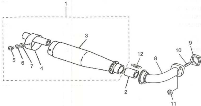
FIG. 4 エキゾースト
